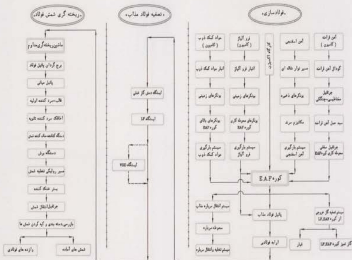
نمودار فرایندی گردش کار واحد فولادسازی
